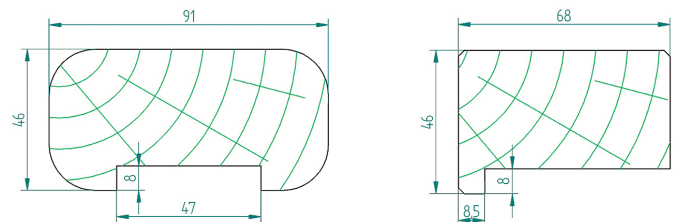
Poteau d'arrêt de cloison
