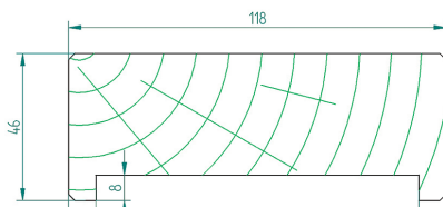
Poteau d'about de cloison
