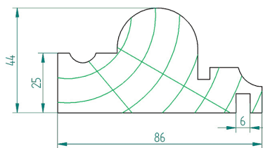
Lisse murale
