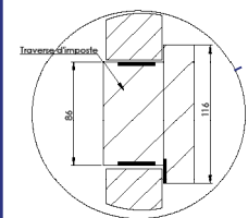
Détail C
