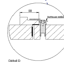
Détail D
